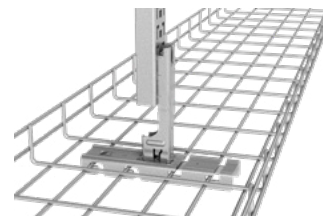
Konsoll for midtoppheng til trådstige.
