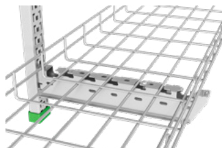
Wibe CLX 3 -konsollen er egnet for både kabelstige, kabelrenne og trådstige.
