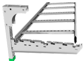
KHZSP-kabelstigen er festet til konsollen for en sikker installasjon.
