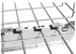
Trådstigene klikkes på plass for sikker installasjon.
