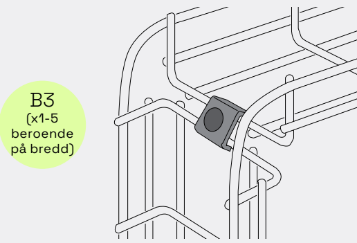
Vertikal avvinkling
