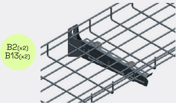
Montage på Konsol 50i
