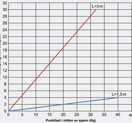
Armaturskena W70/70-200
