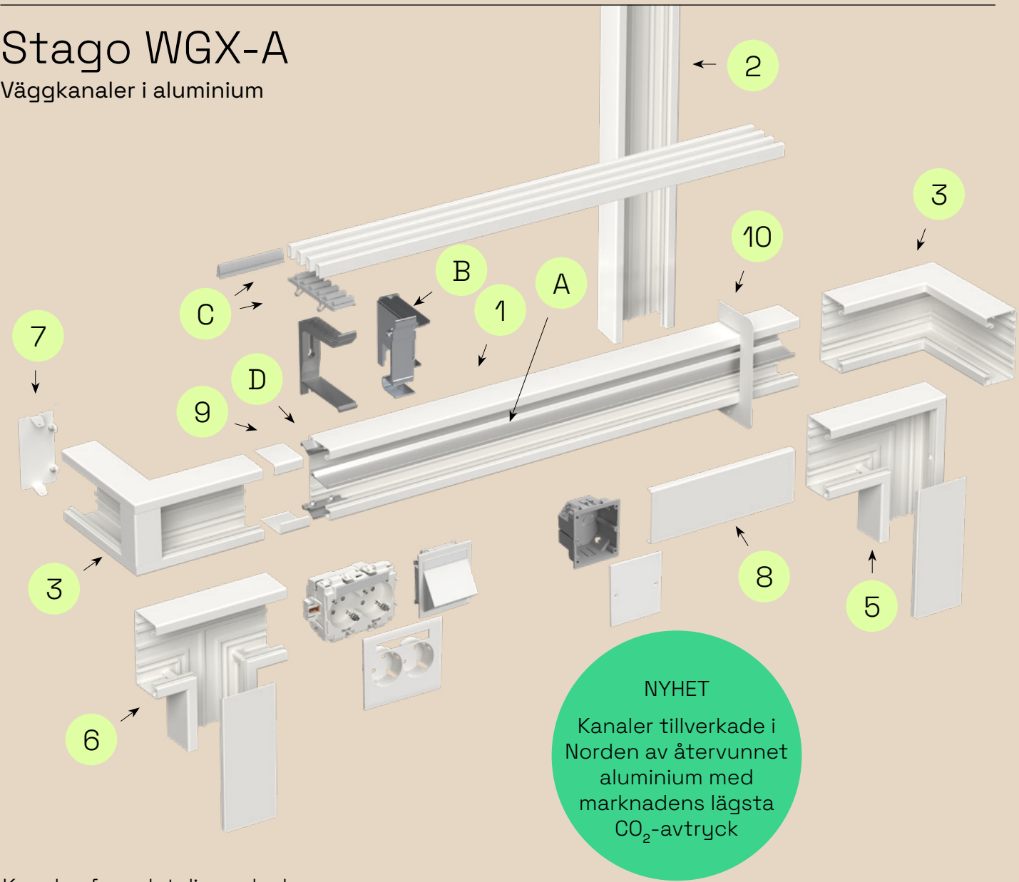
Kanaler, formdetaljer och skarvar m.m.
