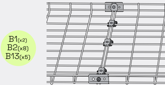
Skarvning trådstege bredd 522-622 mm
