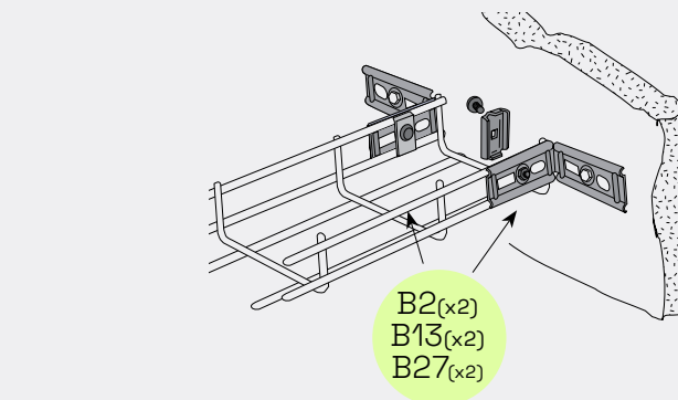
Ändfäste mot vägg
