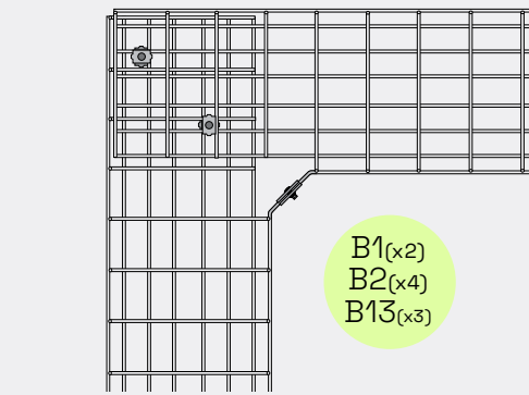
Avvinkling i valfri vinkel
