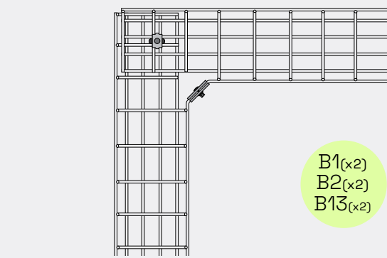
90° avvinkling bredd 522-622 mm
