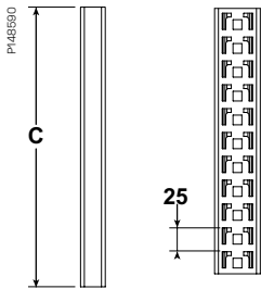
End Plug 28E
